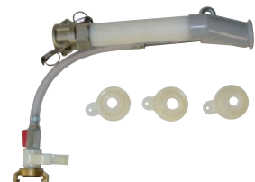
Kit zum Verputzen 1 Putzlanze + 3 Spritzdüsen Ø 8, Ø 12, Ø 16
